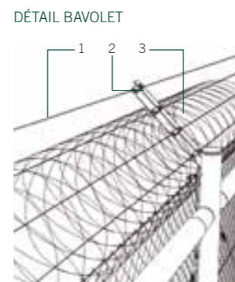
1. BARBELÉ 2. PROFIL SIMPLE EN "T" 3. CONCERTINA
